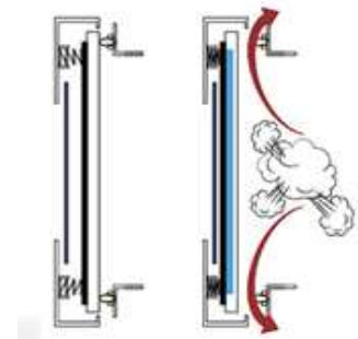
庫内過圧、過熱防止ドア
